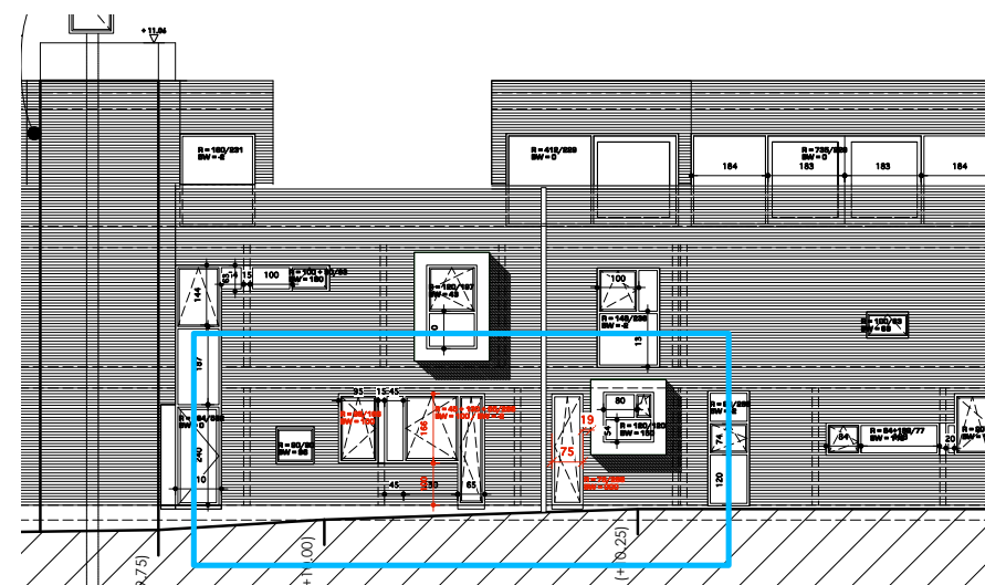
ACHTERGEVEL _ SCHAAL 1/200
