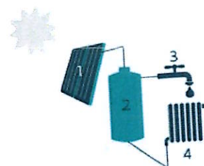
1. Zonnecollector | 2. Opslagvat zonneboiler | 3. Sanitair warm water | 4. Afgifte-element voor ruimteverwarming (radiator)
