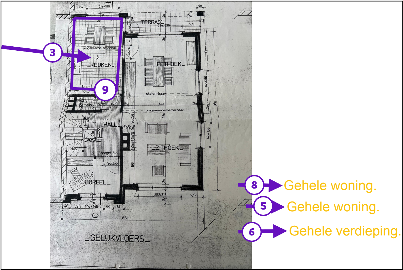
Legende van plan 1.3: Gelijkvloers
