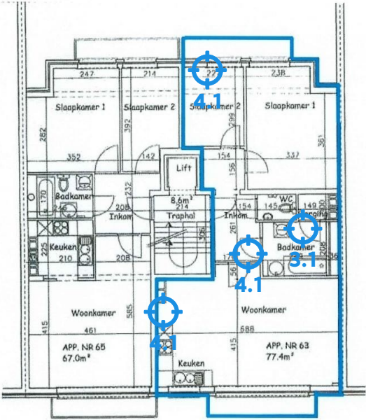
OOSTENDESTRAAAT 2e Verdieping App. 63-65 Schaal 1/100.
